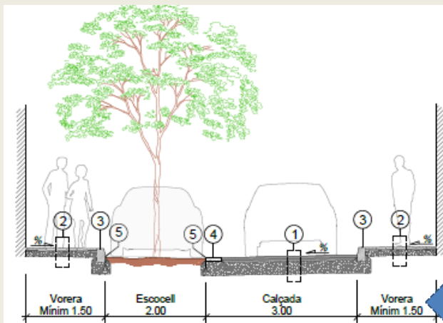
SECCIÓ TIPUS 2a
