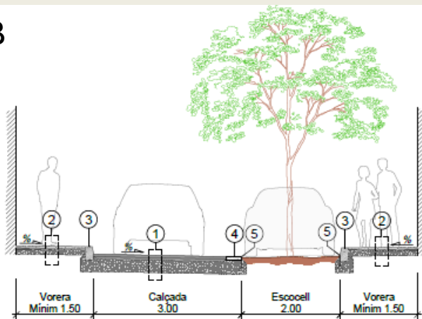
SECCIÓ TIPUS 1a
